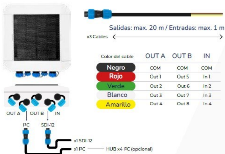
Figura 1. Salidas y entradas dispositivo ATLAS PLUS.
